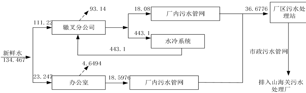
图 2-1 现有工程水平衡图
