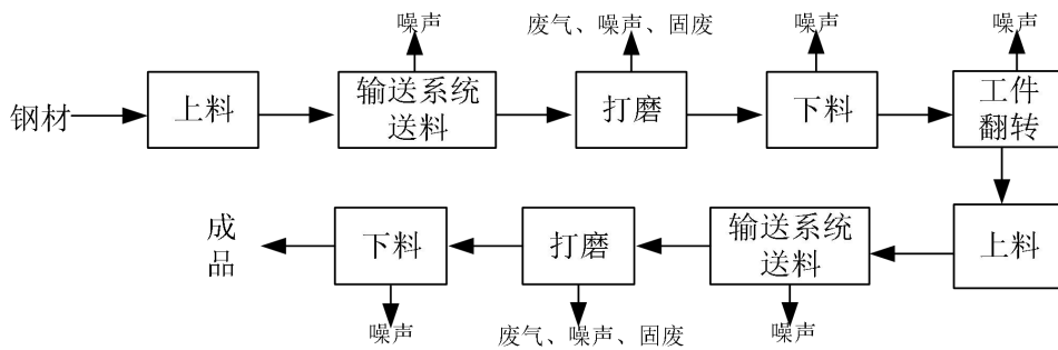
图 2-2 工艺流程图
